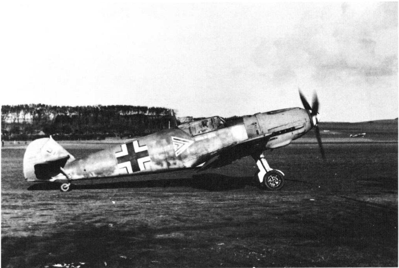
Messerschmitt Bf 109E-4N dowódcy JG 26 „Schlageter” pplk. Adolfa Gallanda, Audembert, Francja, grudzień 1940 roku. Messerschmitt Bf 109E-4N Kommandore JG 26 “Schlageter” Obstl. Adolf Galland, Audembert, France, December 1940 [IWM]
